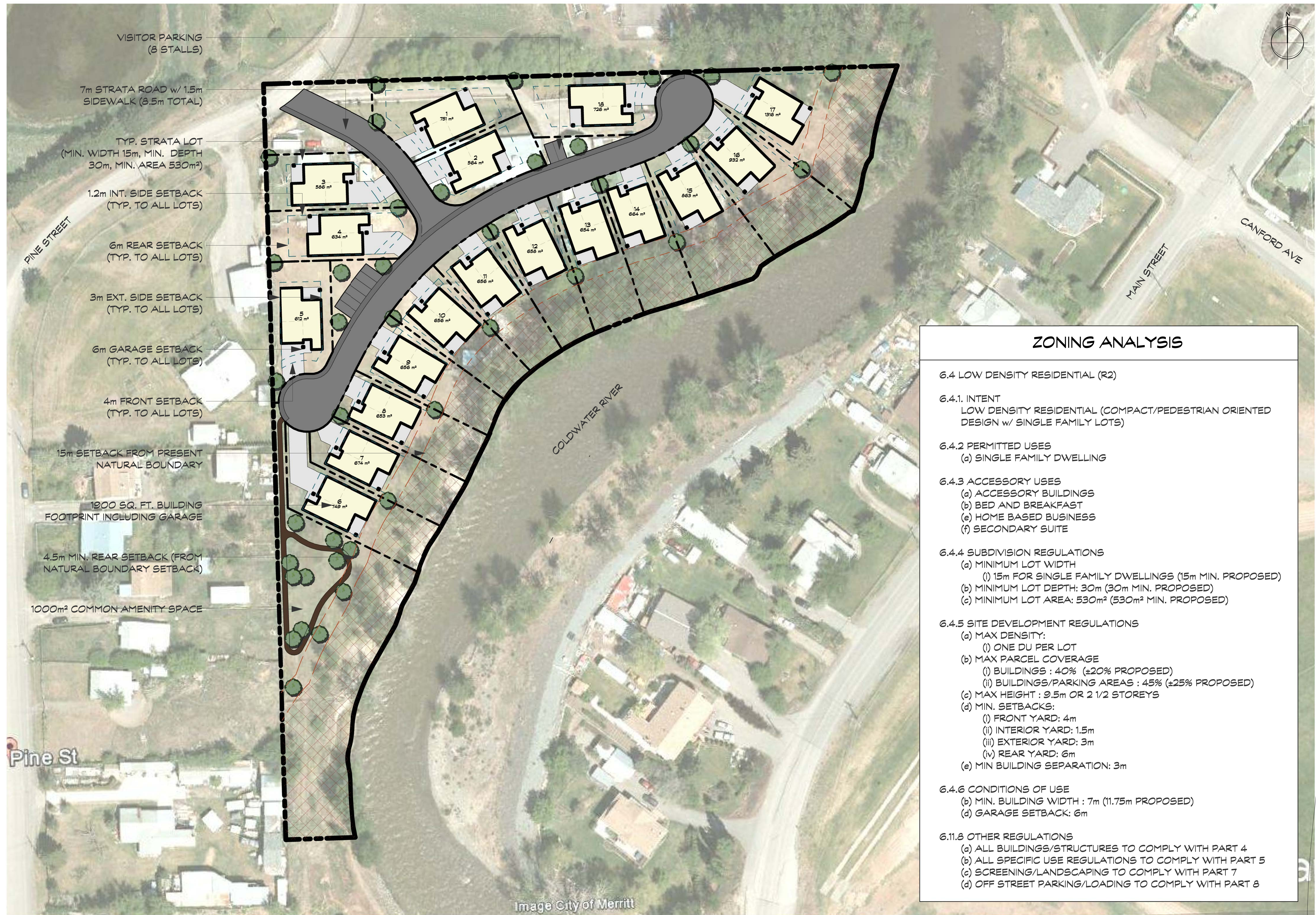
SITE PLAN 1:500
